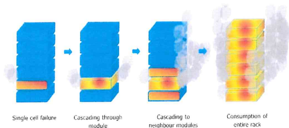
Figura 4 Assenza barriere termiche: Cascading Thermal Runaway
